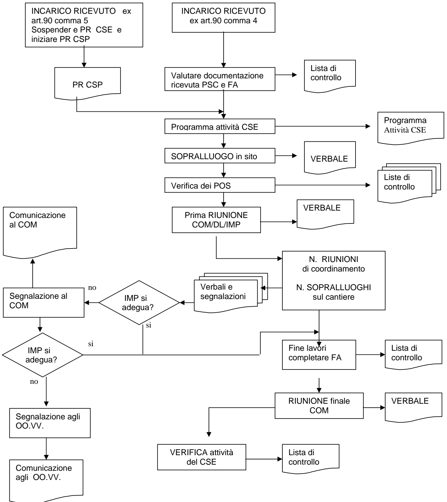
Figura 1 - Diagramma di flusso (CSE)
